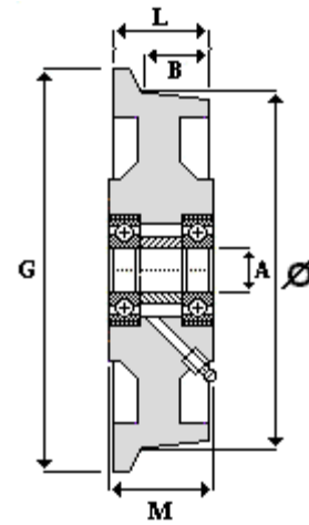
Moyeu à roulements à billes
